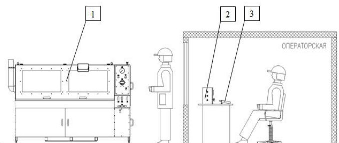
1- бронеканера, 2- блок контроля и регистрации, 3- газоанализатор
